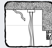
CZ Předšazená záclonová ozdobná lišta - pohled z boku
